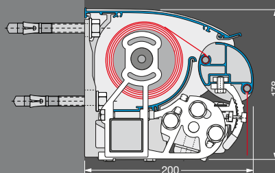
Family Classic Typ Regendach/ Hülse (o. Abb.)
