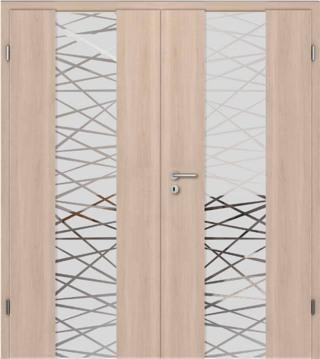
3 MODELL: RY-510-LA5-DA, 2-FLG. , CPL PERA CREME DA GLAS: MIKADO 105-1, Siebdruck-Veredelung MODÈLE: RY-510-LA5-DA, 2 VANTAUX, CPL PERA CRÈME DA VERRE: MIKADO 105-1, Décor par sérigraphie
